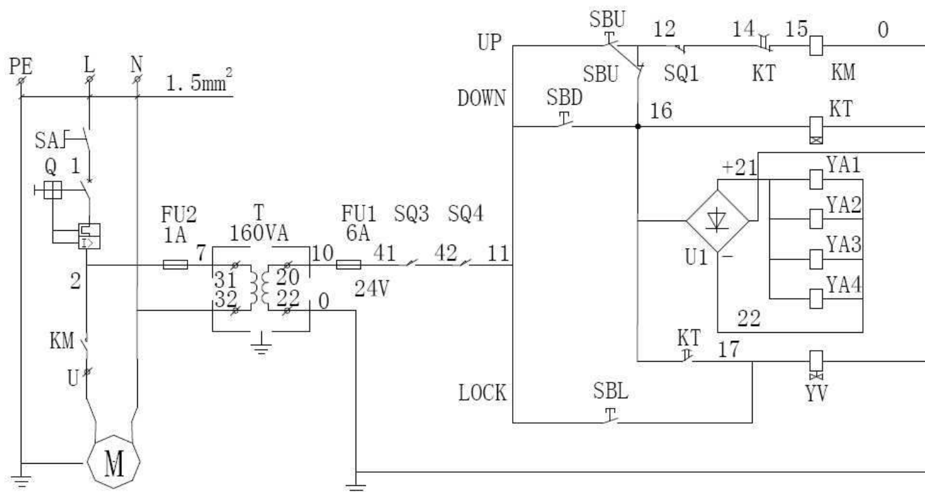
Fig.9a Diagrammi cablaggio monofase Fig.9a Single phase wiring diagrams Fig. 9 a Diagrammes branchement monophasé Abb.9 Diagramme Drehstromverkabelung
