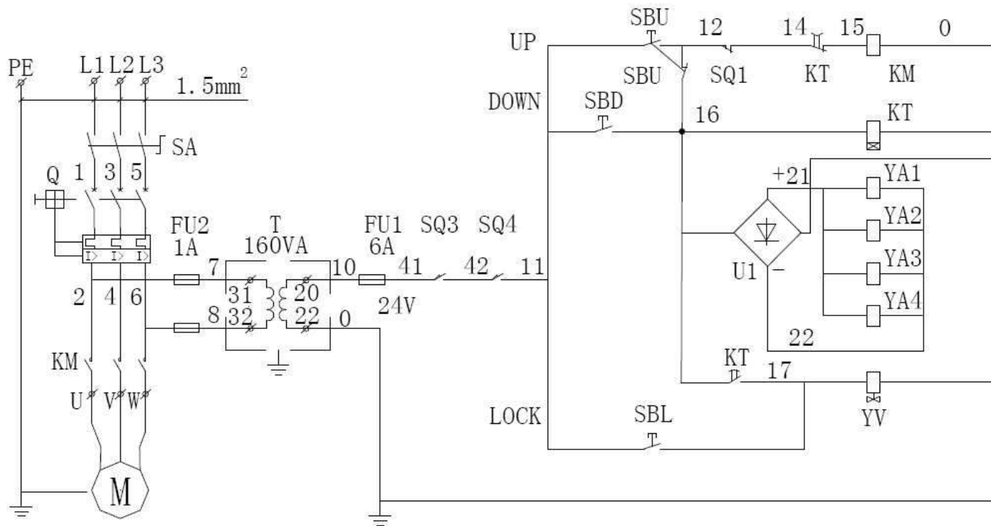
Fig. 9 Diagrammes branchement triphasé
